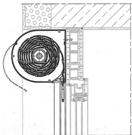
SKO – Rollläden
