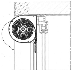
SKO-P – Rollläden
